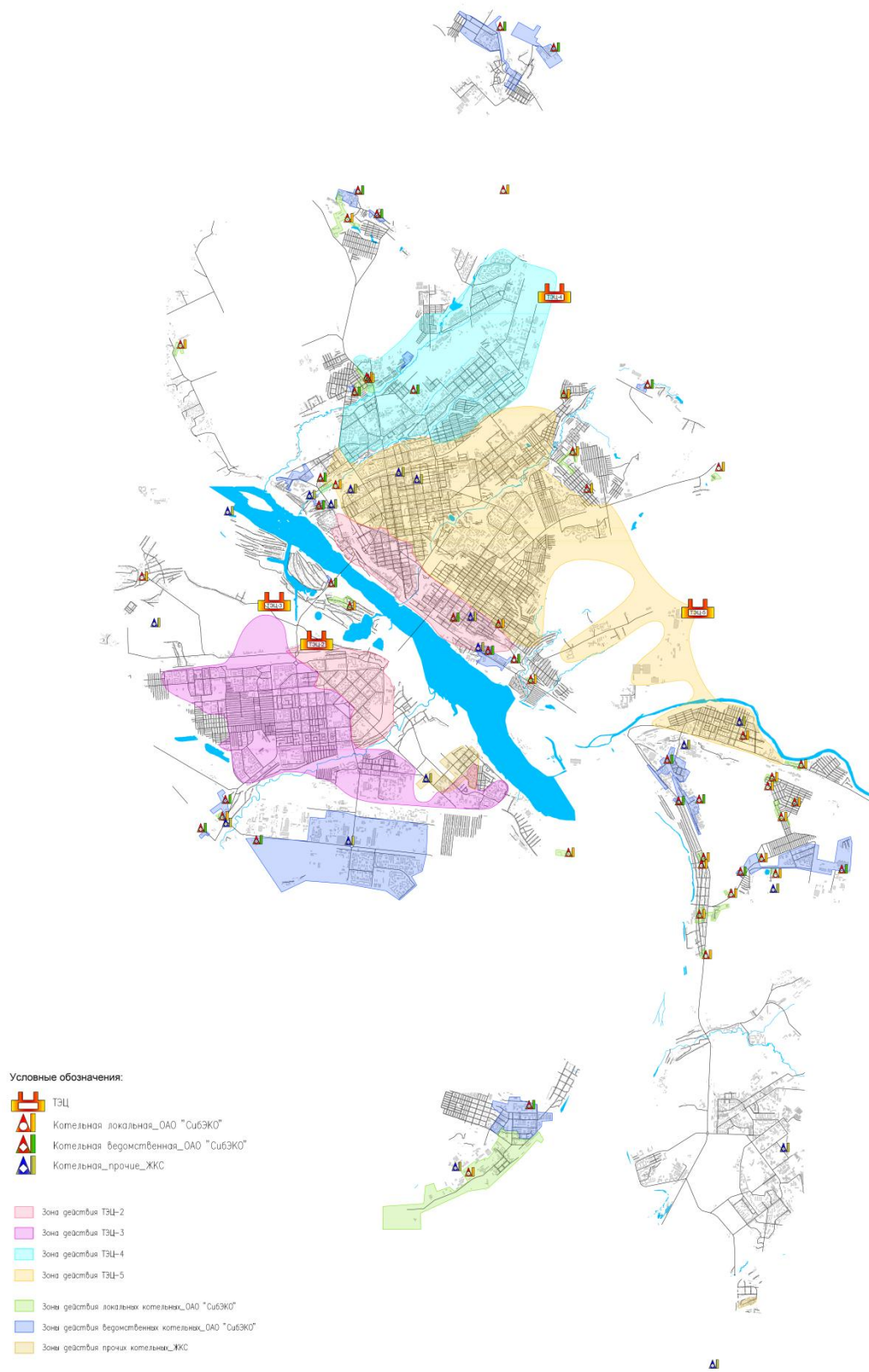
Рисунок 3.1 – Зоны действия тепломагистралей от ТЭЦ-2, ТЭЦ-3, ТЭЦ-4, ТЭЦ -5 и крупных котельных
