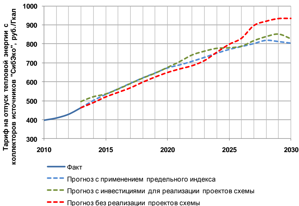
Рисунок 8.7. Динамика изменения тарифа на отпуск тепловой энергии от энергоисточников ОАО «СИБЭКО», определенная для различных сценариев
