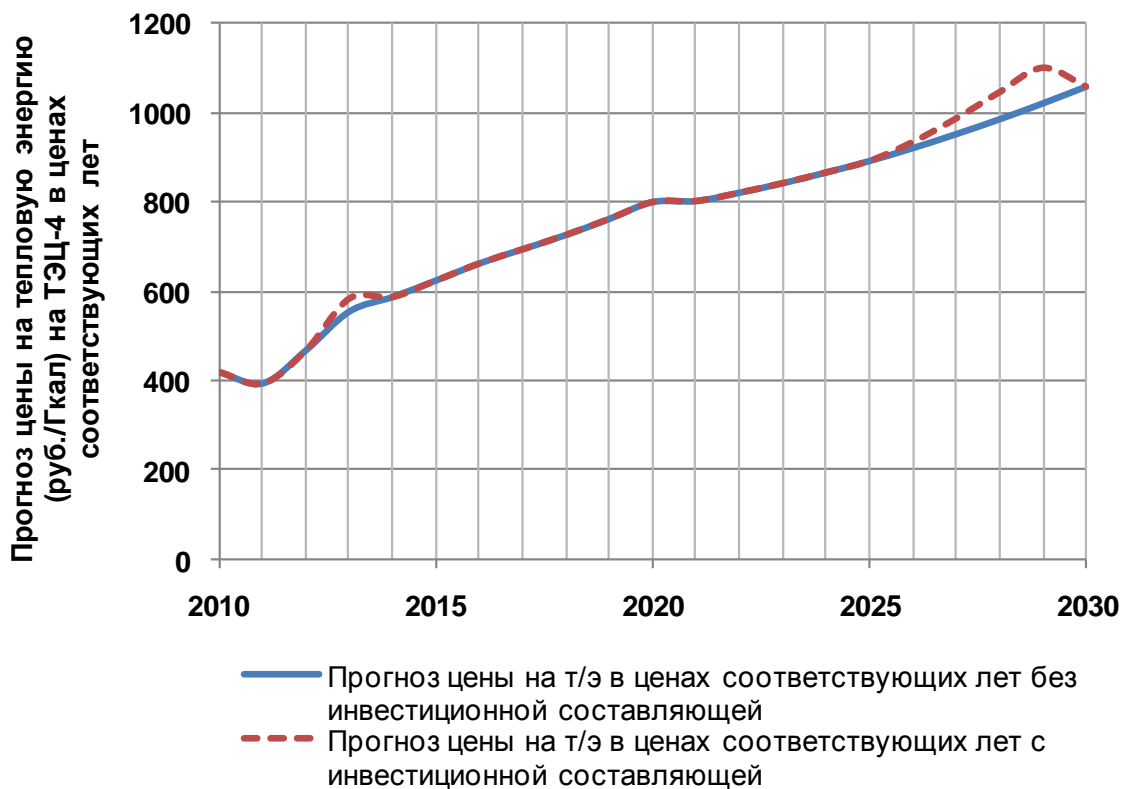
Рисунок 8.3 - Прогноз цены на тепловую энергию, отпущенную с коллекторов ТЭЦ-4 (в ценах соответствующих лет)
