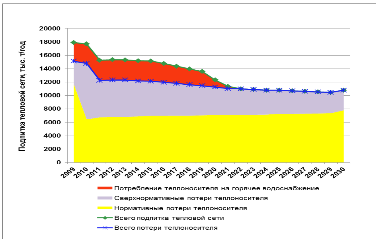
Рисунок 4.1 - Прогноз подпитки тепловой сети в зонах действия источников тепловой энергии города Новосибирска
