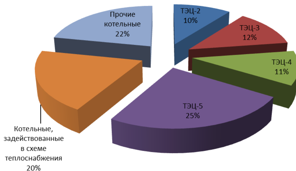
Рисунок 10.2 – Распределение присоединенной нагрузки между энергоисточниками города Новосибирска в 2015 году
