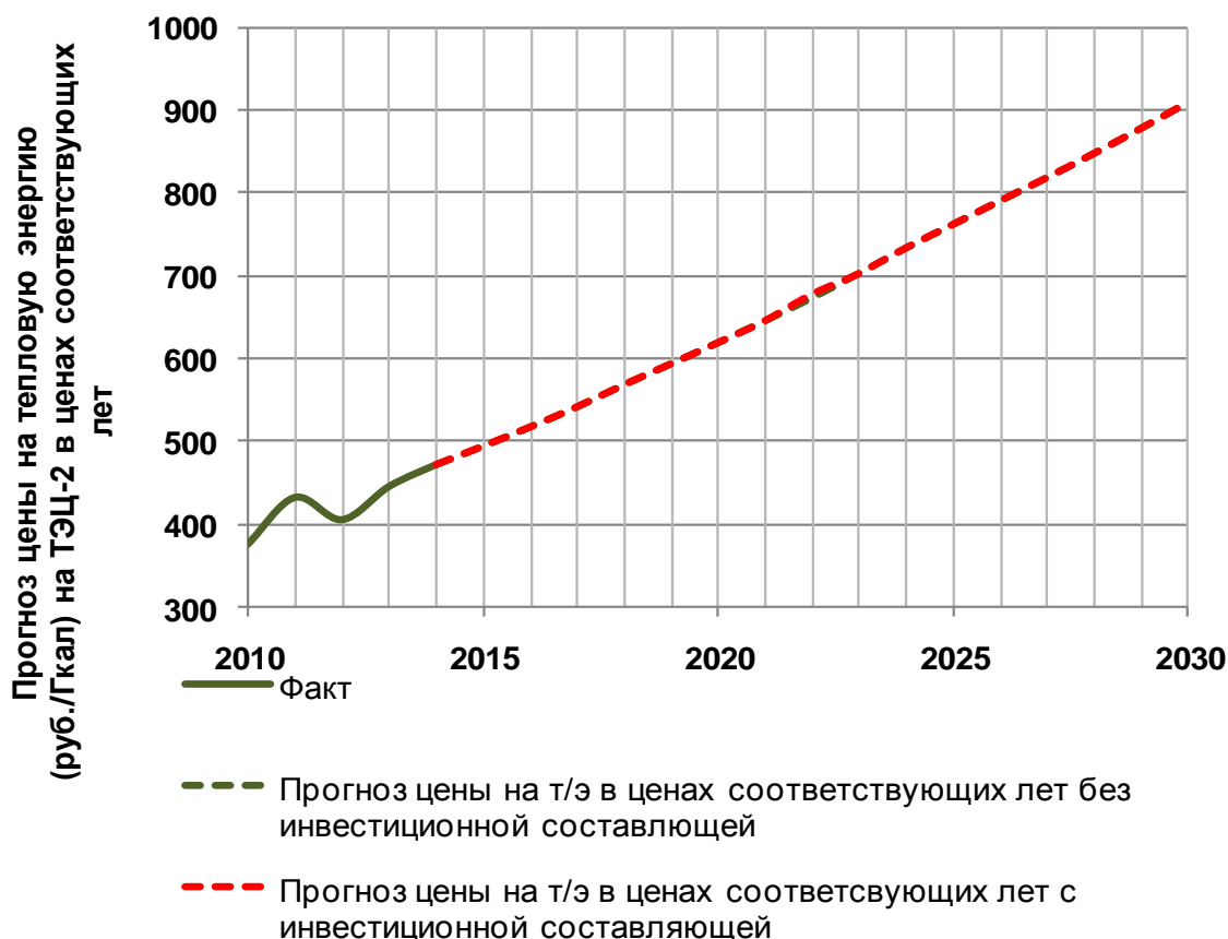
Рисунок 8.1 - Прогноз цены на тепловую энергию, отпущенную с коллекторов ТЭЦ-2 (в ценах соответствующих лет)
