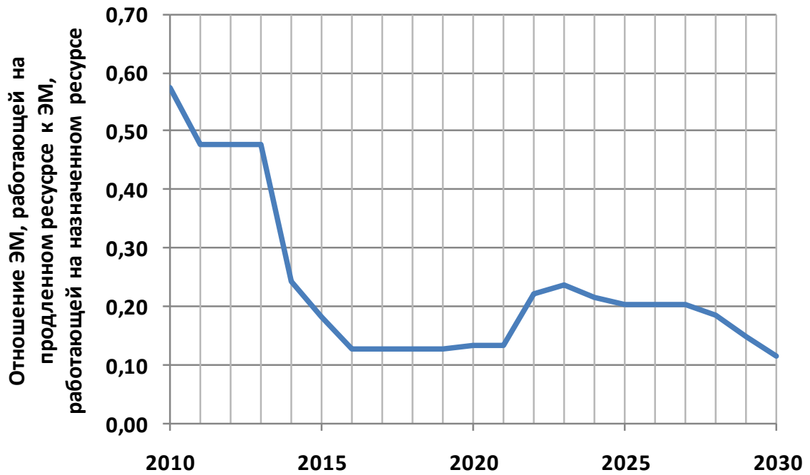
Рисунок 1.4 – Изменение соотношения между мощностью, работающей на продленном и нормативном ресурсе, для ТЭЦ г. Новосибирска
