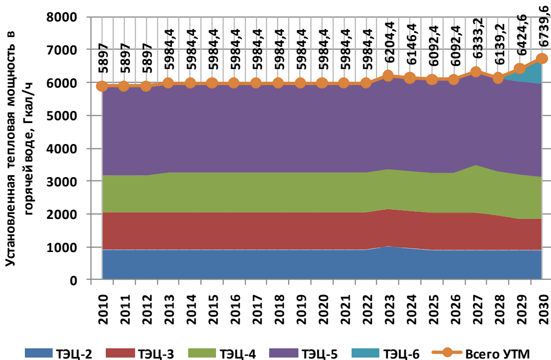
Рисунок 1.6. Динамика изменения установленной тепловой мощности в горячей воде электростанций г. Новосибирска (с выделением каждой станции)
