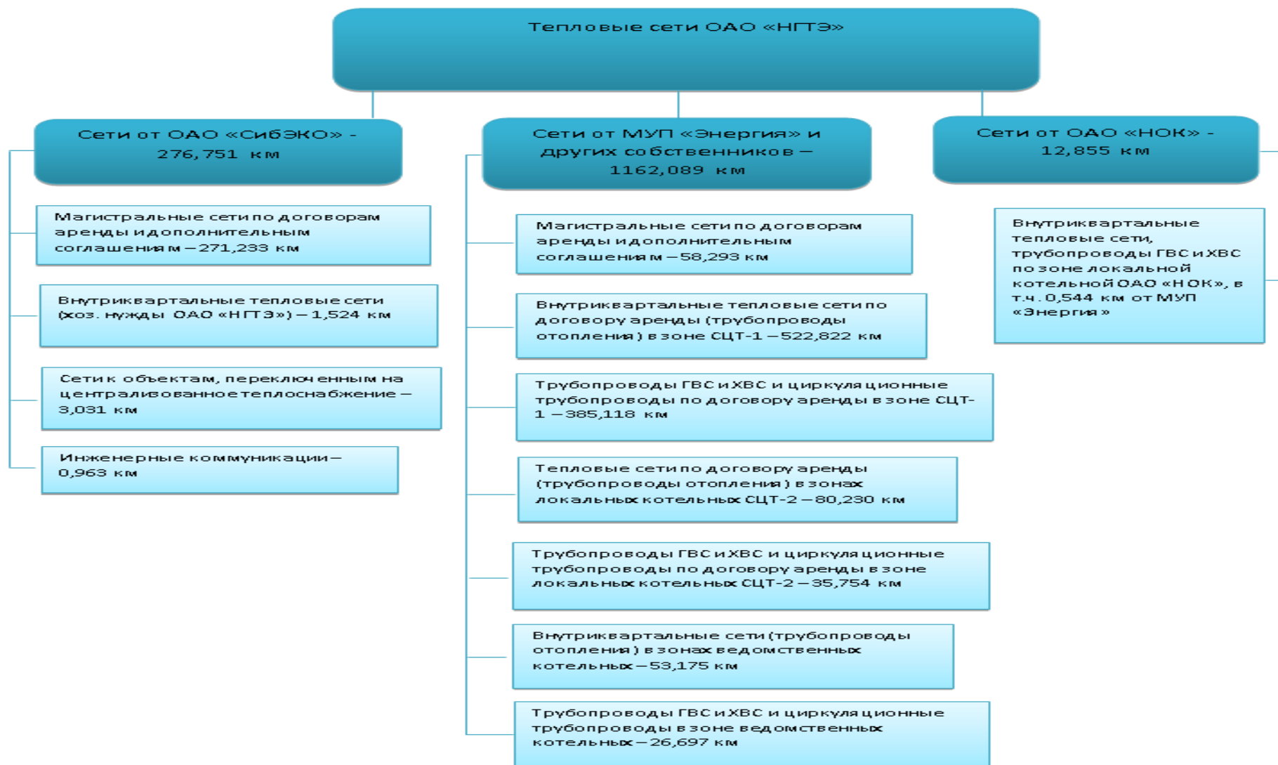
Рисунок 1.3 - Структура тепловых сетей ОАО «НПТЭ»
