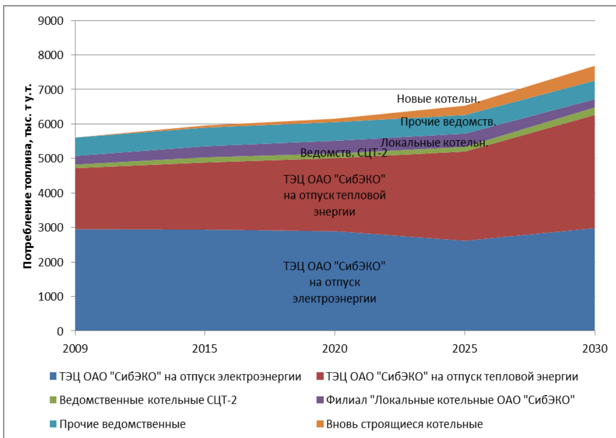
Рисунок 7.1 – Прогнозное потребление топлива энергоисточниками города Новосибирска
