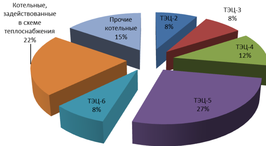
Рисунок 10.5 – Распределение присоединенной нагрузки между энергоисточниками города Новосибирска в 2030 году
