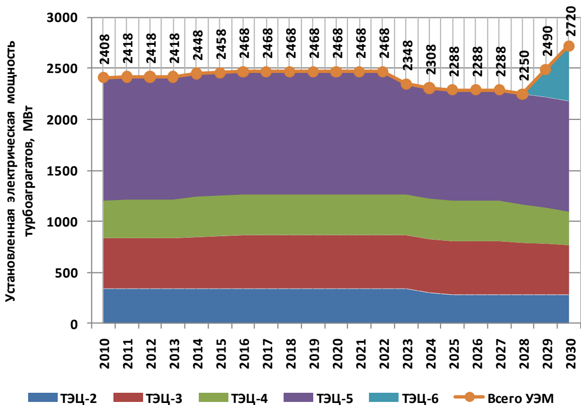
Рисунок 1.5. Динамика изменения установленной электрической мощности электростанций г. Новосибирска (с выделением каждой станции)
