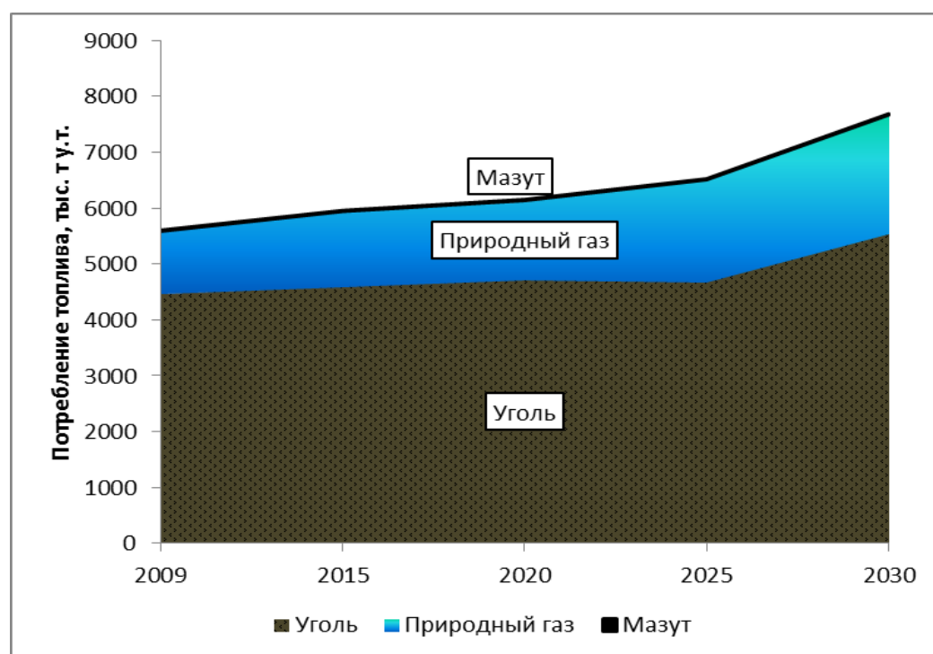
Рисунок 7.2 – Изменение потребления топлива энергоисточниками города Новосибирска по видам топлива
