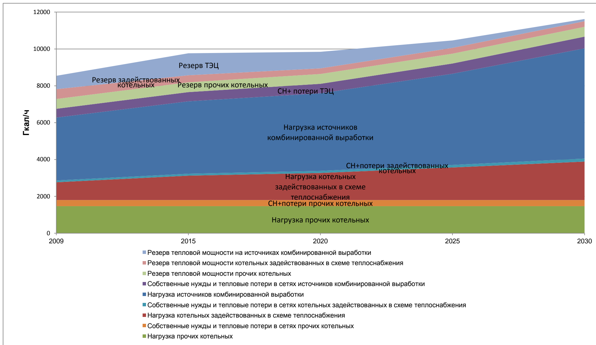
Рисунок 3.7 - Структура тепловых нагрузок и резервов тепловой мощности энергоисточников города Новосибирска
