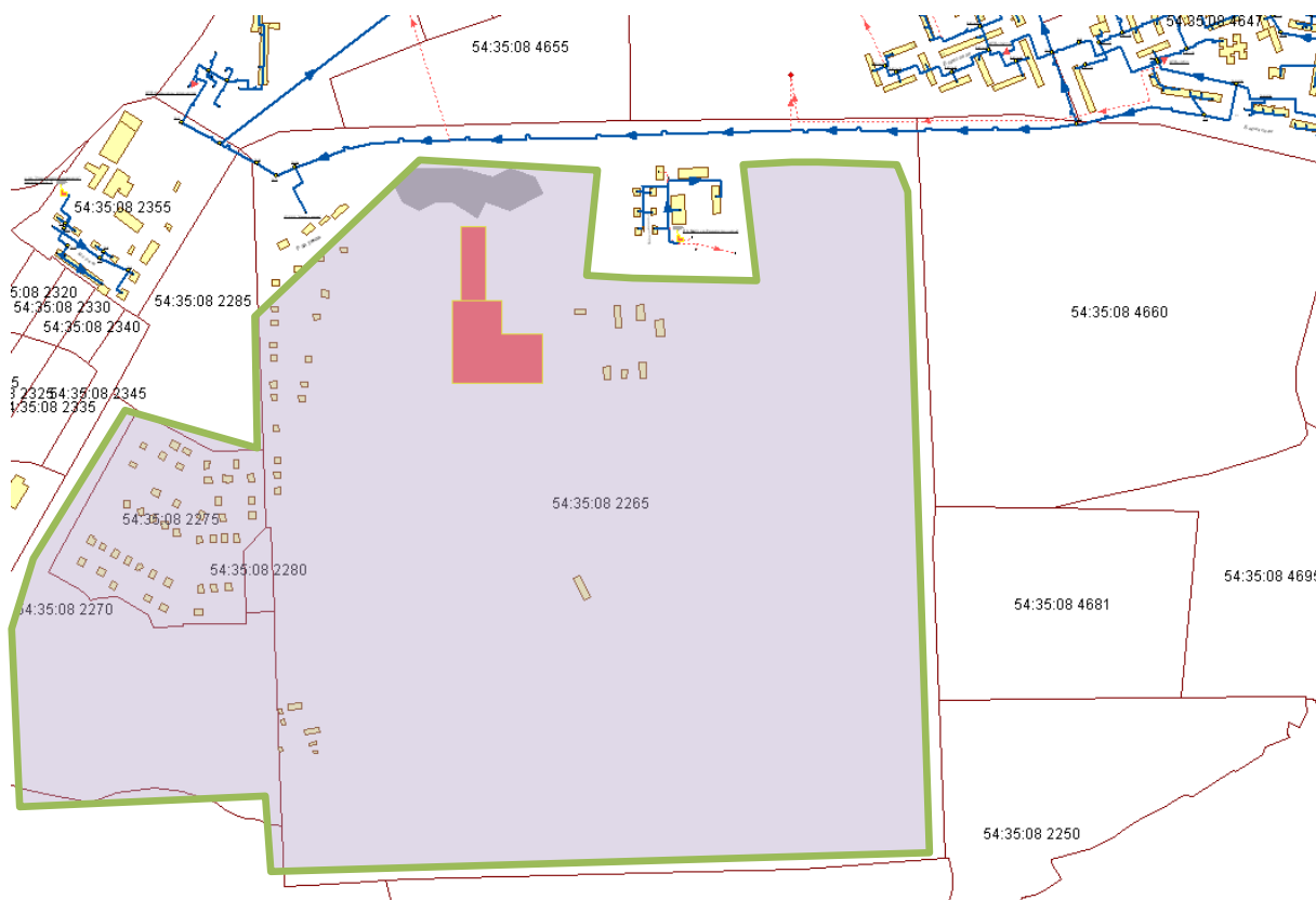
Рисунок 3.6 - Зона действия предлагаемой к строительству котельной «Березовая»
