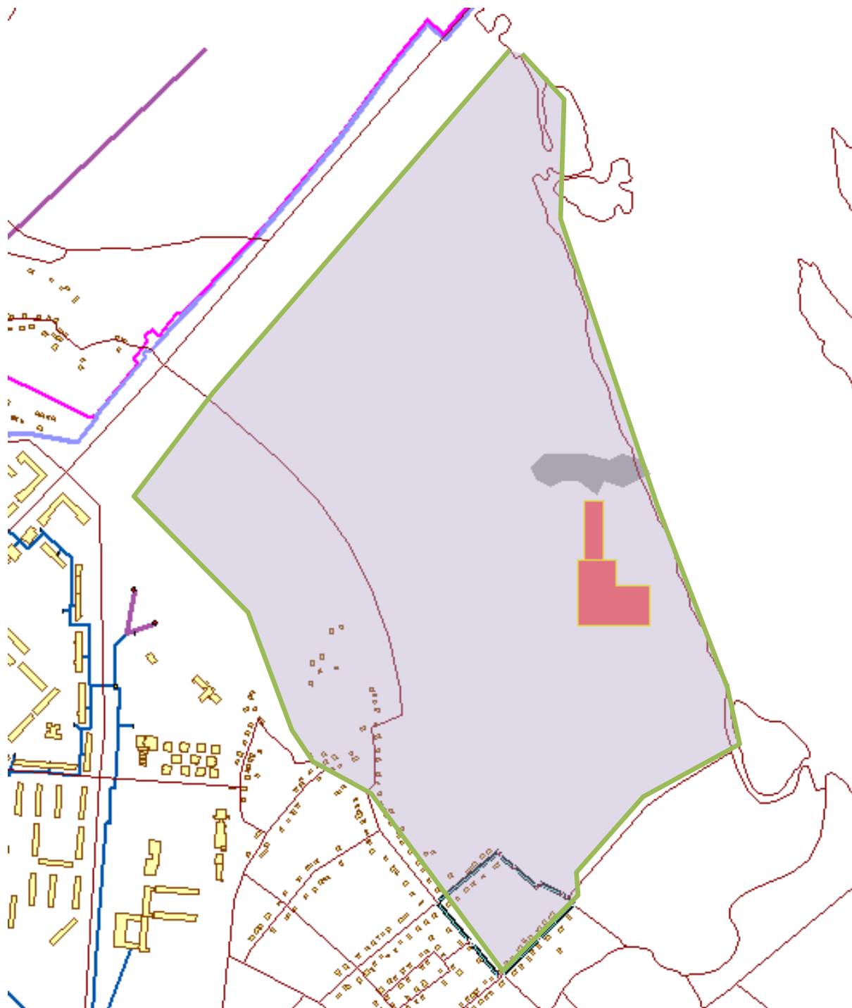
Рисунок 3.3 - Зона действия предлагаемой к строительству котельной «Спортивная»
