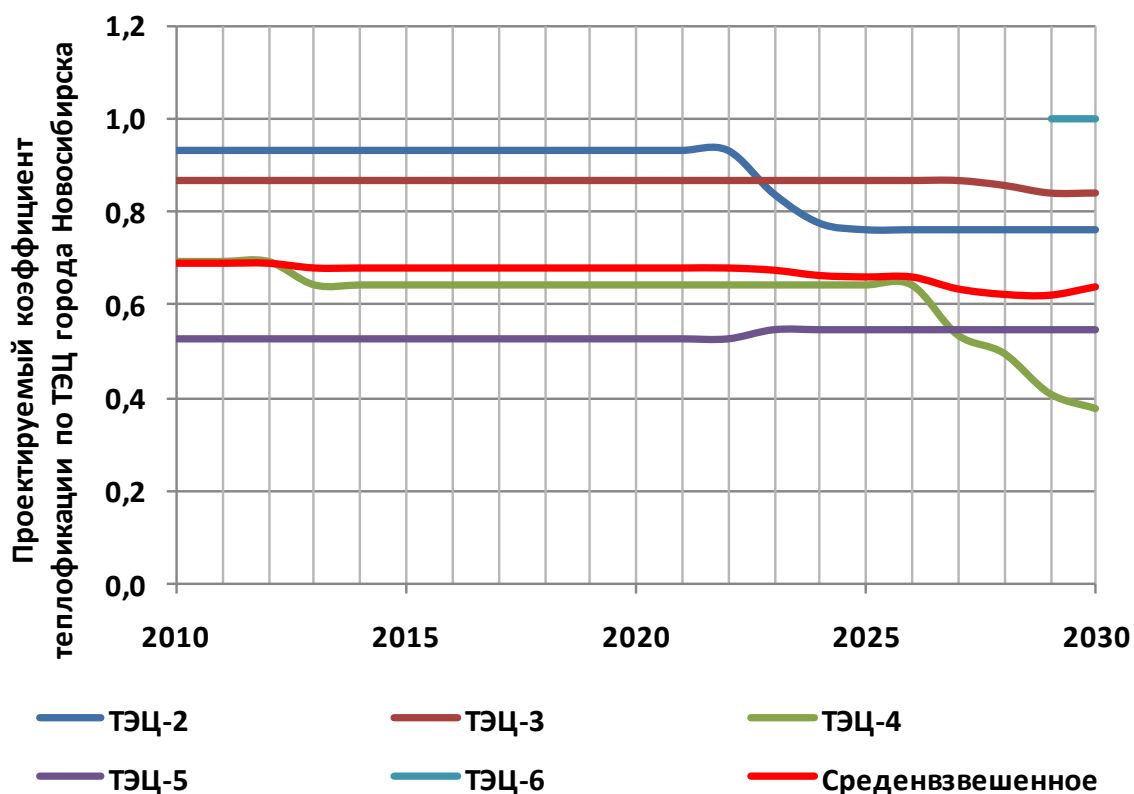
Рисунок 1.7 – Изменение проектируемого коэффициента теплофикации ТЭЦ г. Новосибирска
