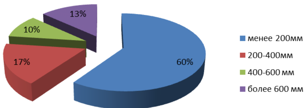
Рисунок 1.2 - Распределение протяженности тепловых сетей города Новосибирска по условным диаметрам на конец 2009 года
